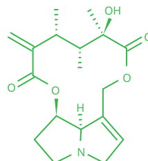
Senecivernine
