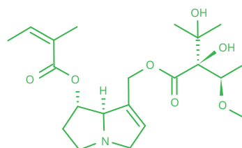
Lasiocarpine
