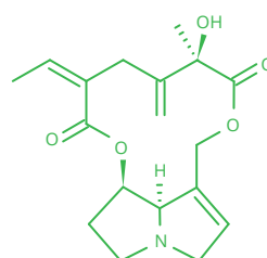
Seneciophylline
