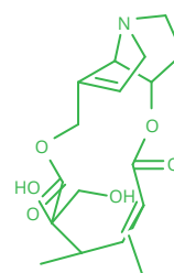
Retrorsine
