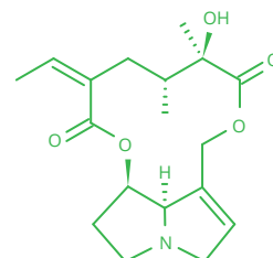
Senecionine
