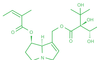
Echimidine
