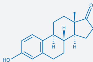
Estrone (E1)
