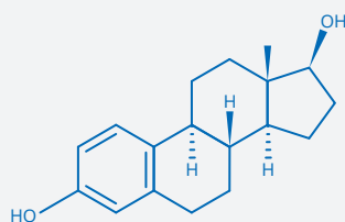
Estradiol (E2)
